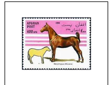
Merychippus (Miocène)
