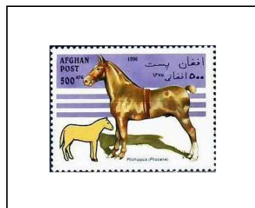
Pliochippus (Pliocène)
