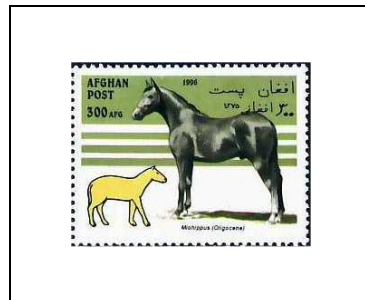
Miochippus (Oligocène)
