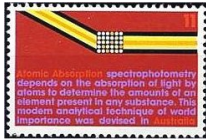
Pollution atomique
