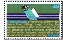
Océanographie
