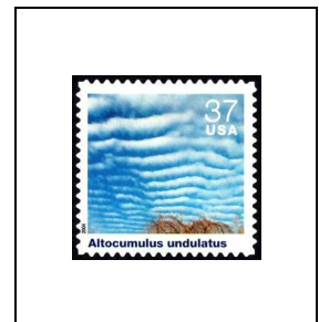
Alto cumulus undulatus
