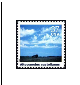
Alto cumulus castellanus
