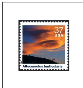
Alto cumulus lenticularis
