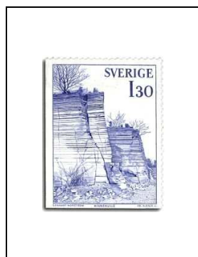
Le roc de Rodstenskleven
