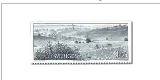
Les collines de Brösarp en Scanie
